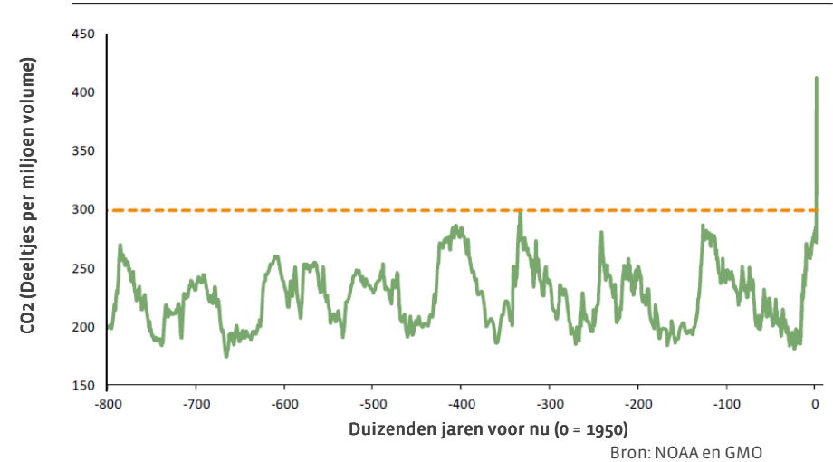
Koolstofdioxide concentratie in de atmosfeer
